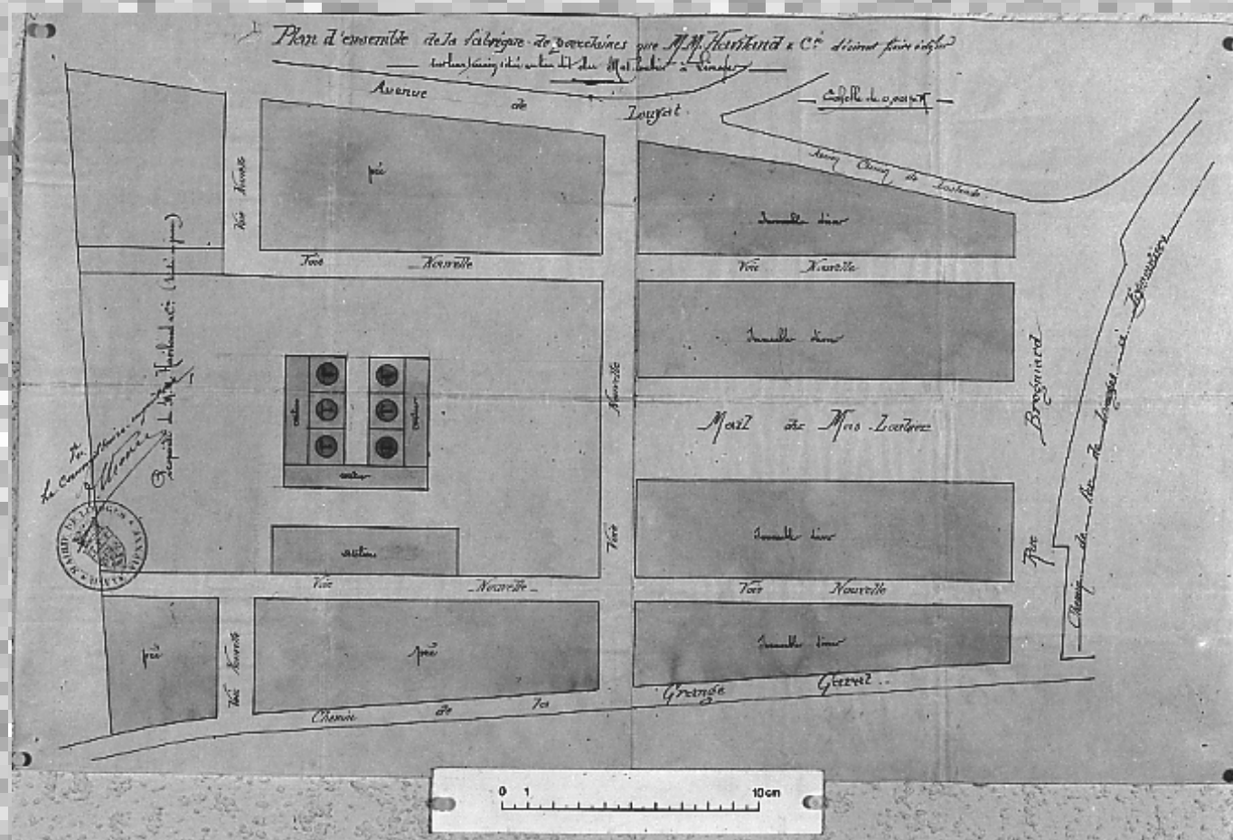
Plan d'ensemble de la fabrique de porcelaines que MM. Haviland & Cie désirent faire édifier sur leur terrain situé au lieu-dit du Mas-Loubier à Limoges. Plan, 1 : 1000, 48 x 29 cm, 1895. AD Haute-Vienne : 5 M 51.
