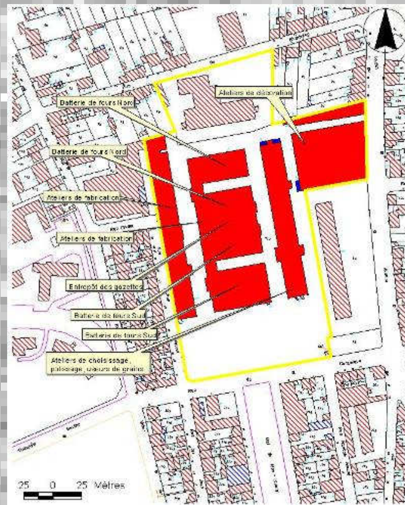
Plan masse de l'usine
